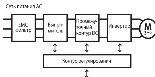
Рис. 79 Основные блоки, составляющие преобразователь частоты
