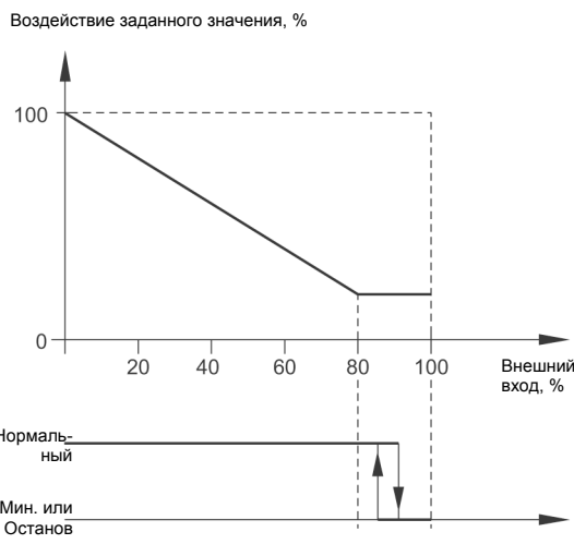
Рис. 58. Обратная функция с остановом и обратная функция с минимумом
