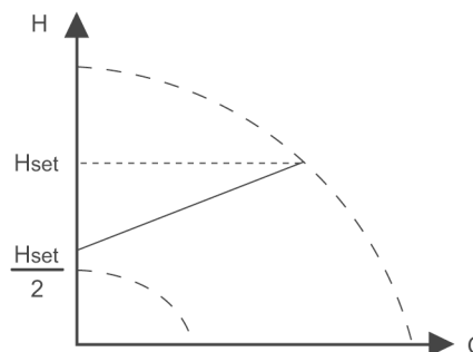
Рис. 37. Пропорциональное давление
