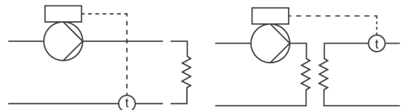
Рис. 42. Постоянная температура
