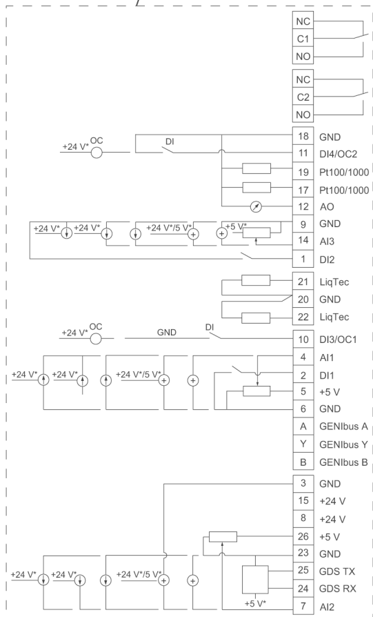
Рис. 77. Соединительные клеммы, FM 300 (на заказ)
