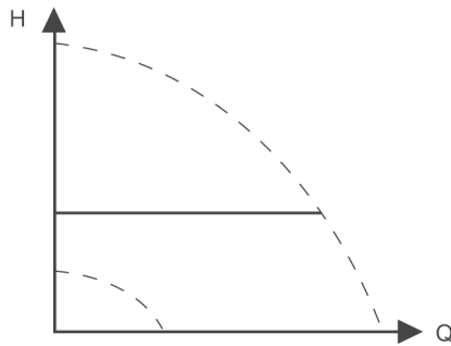
Рис. 39. Постоянное давление
