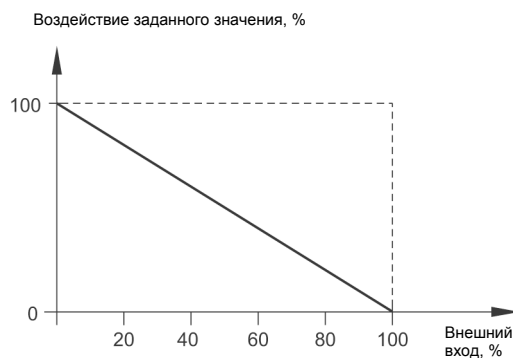
Рис. 57. Обратная функция
